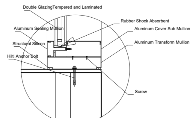
Detail - 10 Scale: 1/5
